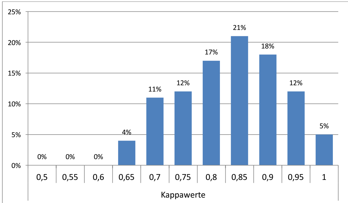
Abb. 3.3.2.1: Verteilung der Untersuchungsübereinstimmung (Kappa) bei der Kalibrierung (n=482): Ein Kappa-Wert von 1 bedeutet ideale Übereinstimmung zwischen kalibrierter Person und Referenzperson, ein Kappa-Wert von 0 keinerlei Übereinstimmung.
